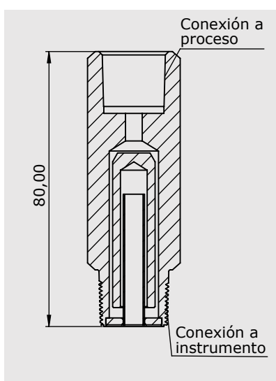
Fig 5. Dimensiones modelo 095.
