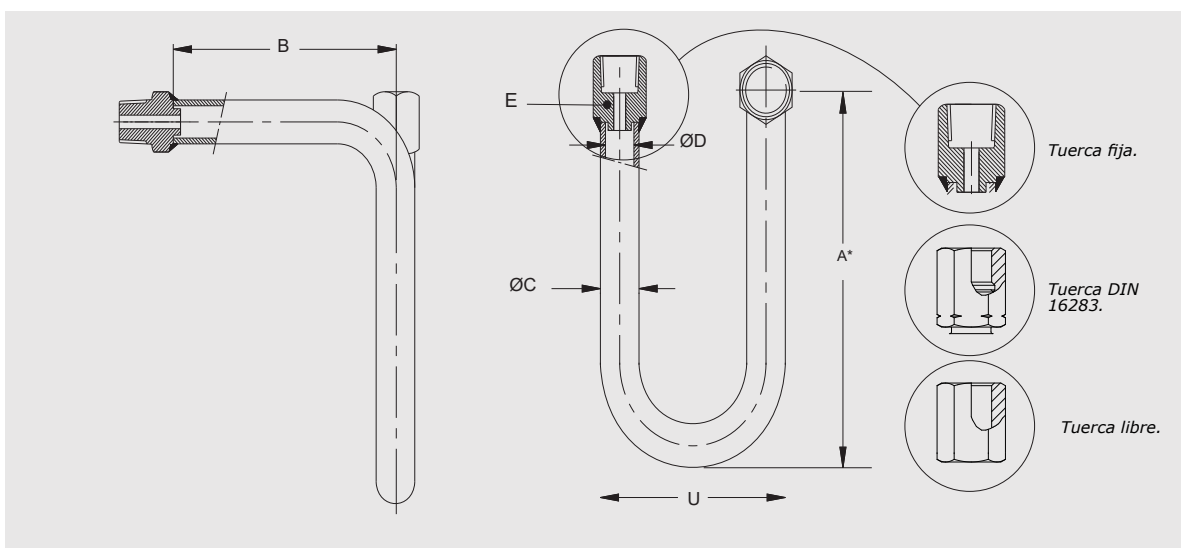
Fig 4. Dimensiones modelo 092.
