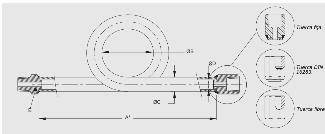
Fig 2. Dimensiones modelo 090.
