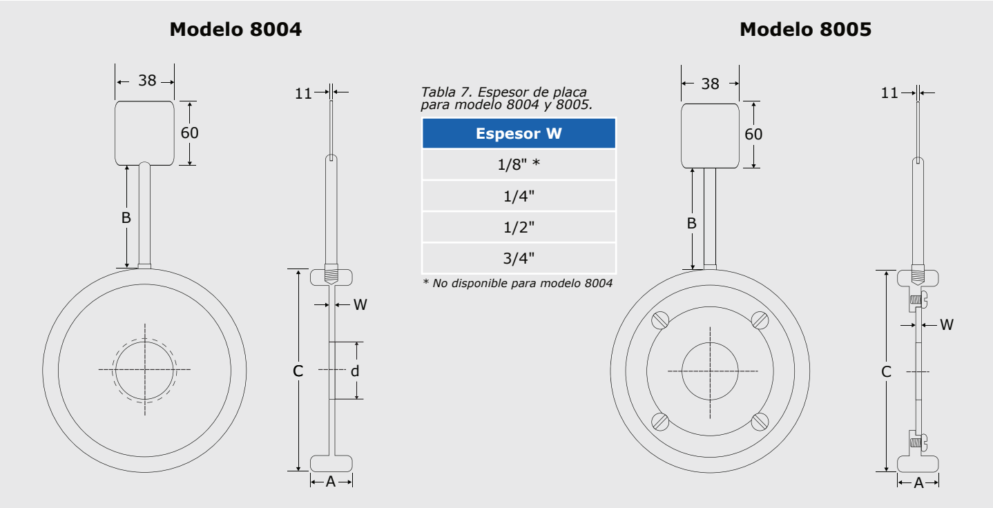
Fig 13. Dimensiones en mm de placa orificio modelo 8004 y 8005.
