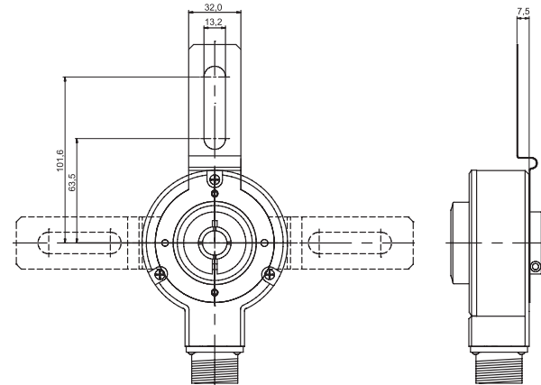
Lâmina grande - Fixação tipo 3.
